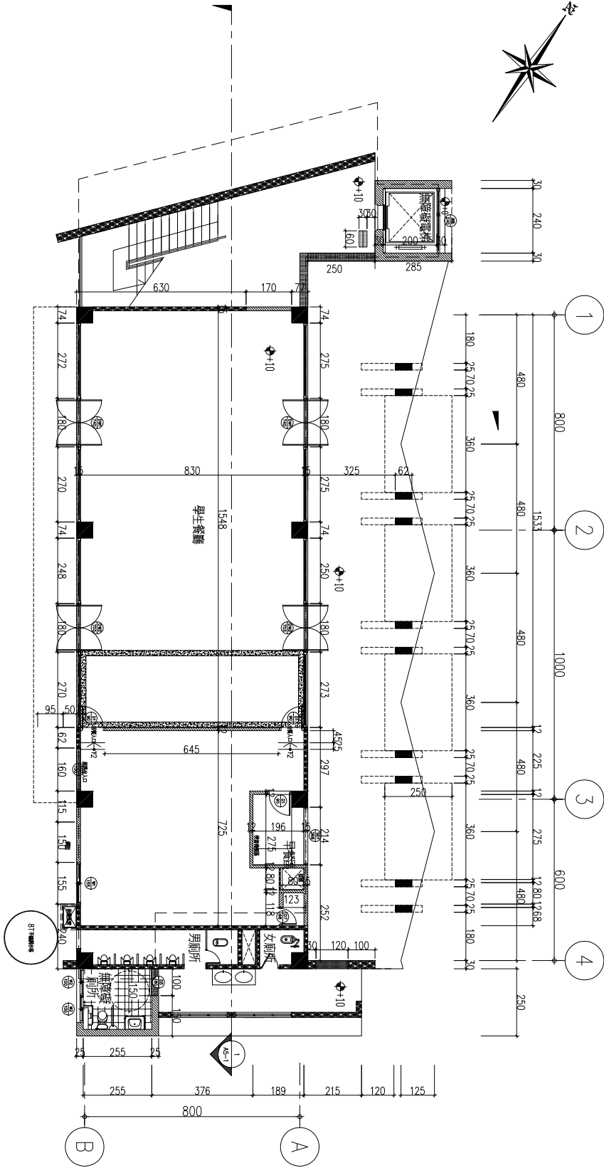
壹層平面圖 S:1/100
