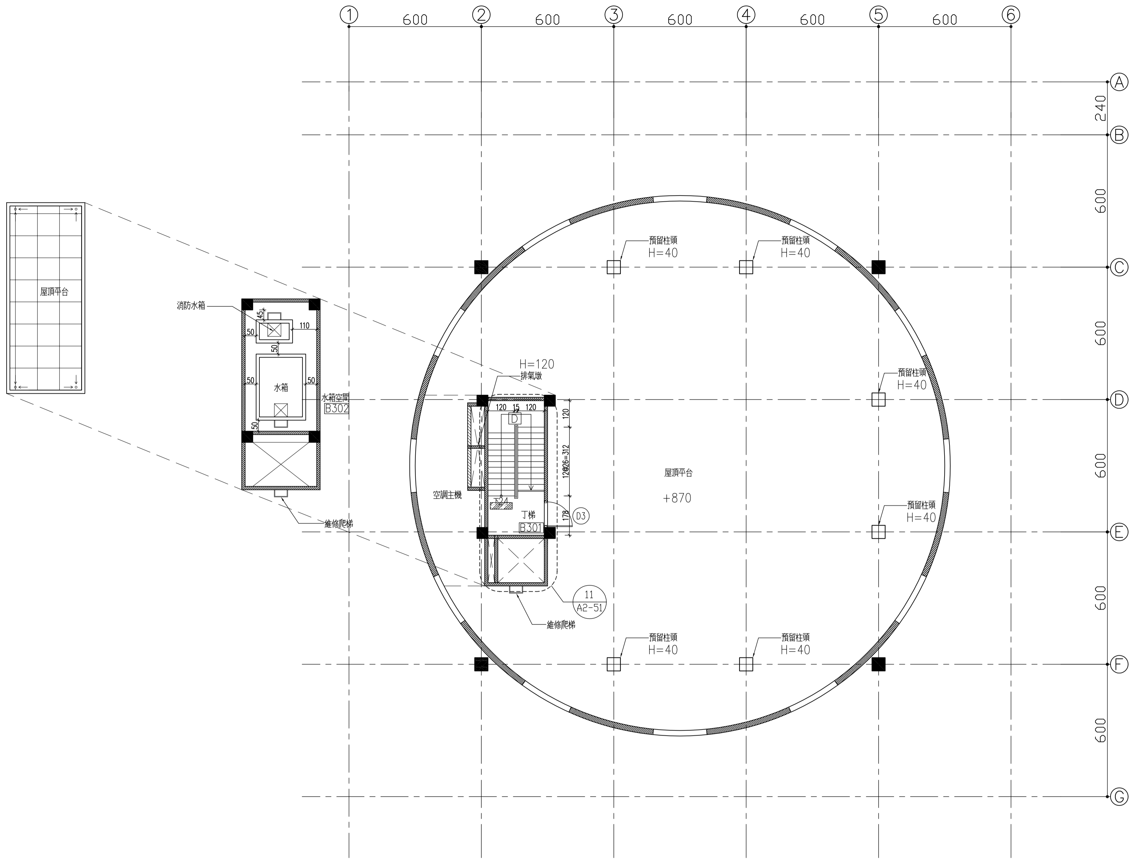
1 生活設施棟屋突一層平面圖 A2-07 A1 S:1/100 A3 S:1/200 U:CM
